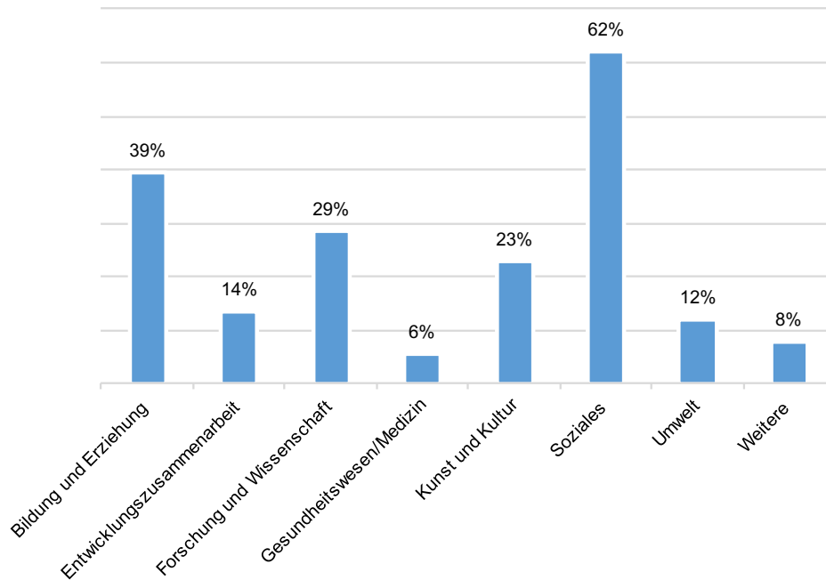
Grafik 3: Förderbereiche
